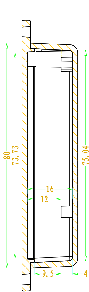
SEC A-A
