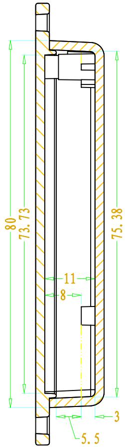
SEC A-A
